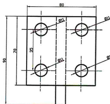
Kronšteins. Skats C.
