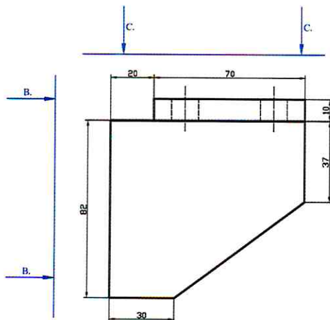
Kronšteins. Skats A.
