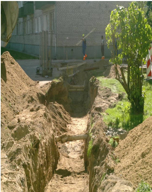
Vienkāršotā siltumtrases rekonstrukcija no Lidotāju ielas 20 līdz Lidotāju ielai 22, Saldus ielai 1, 3, Ventspilī
