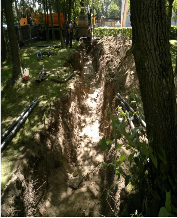
Vienkāršotā siltumtrases rekonstrukcija no Lidotāju ielas 11 līdz Lidotāju ielai 13, Ventspilī
