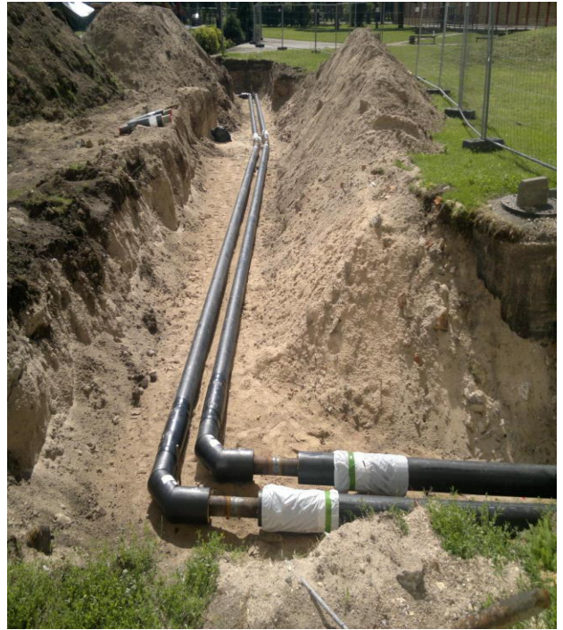
Siltumtrase rekonstrukcija starp ēkām Saules ielā Nr.106, Nr.114 un Nr.116, Ventspilī
