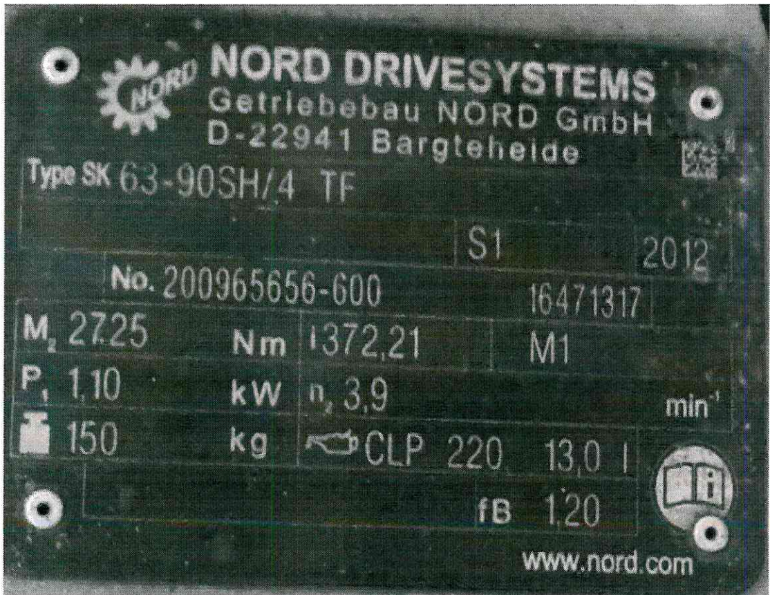
7) Reduktors Nr. 7
